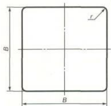
Рисунок Д.5 - Размеры квадратных знаков
